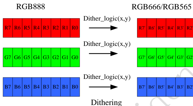
Fig. 22-17 LCDC Dithering
