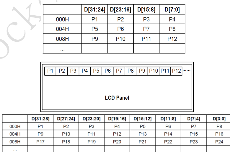
Fig. 22-4LCDC Win1 Palette (8bpp/4bpp)
