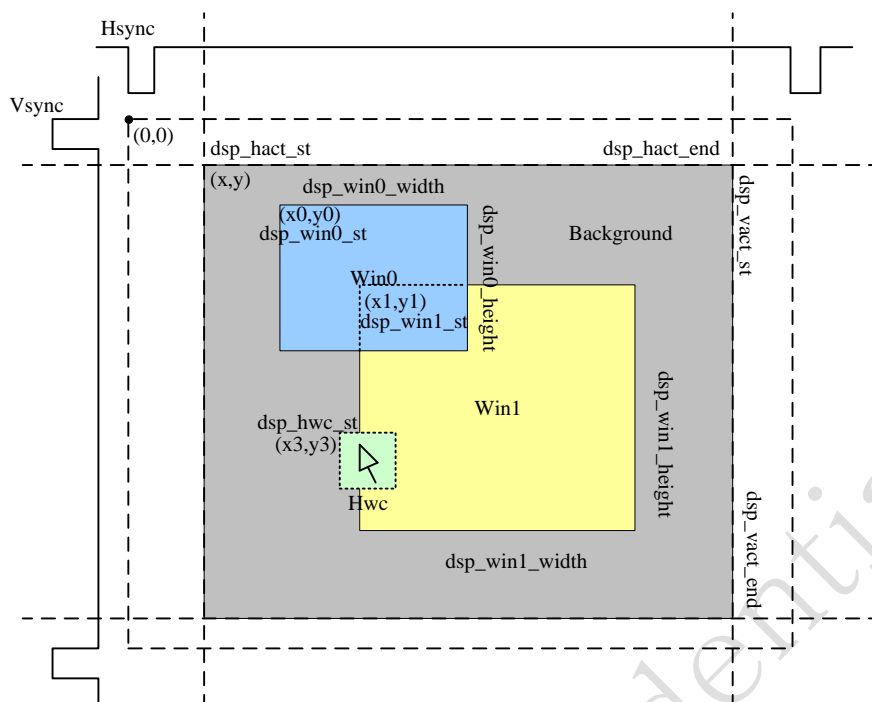
Fig. 22-13LCDC Overlay Display
