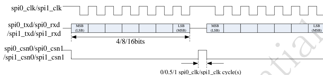
Fig. 35-4 SPI Format (SCPH=0 SCPOL=1)
