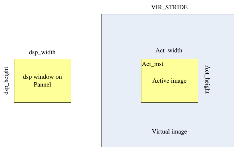
Fig. 22-6LCDC Virtual Display Mode
