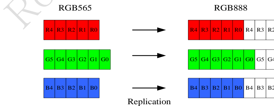
Fig. 22-16LCD Replicaiton
