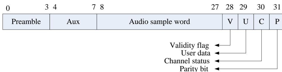
Fig. 30-3SPDIF Sub-frame Format
