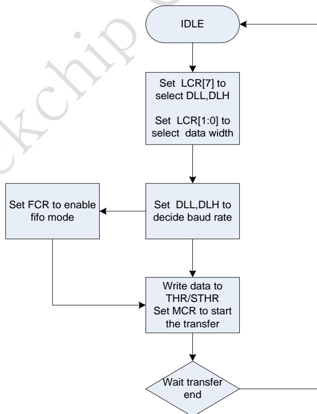
Fig. 36-8UART fifo mode
