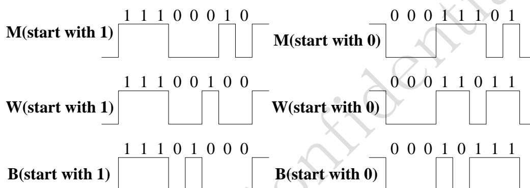
Fig. 30-5 SPDIF Preamble
