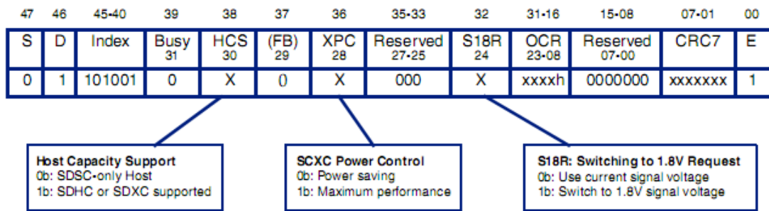
Fig. 1-13 ACMD41 Argument
