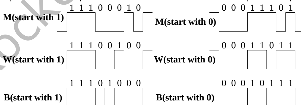
Fig. 14-5 SPDIF Preamble
