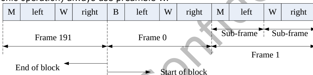
Fig. 14-2 SPDIF Frame Format
