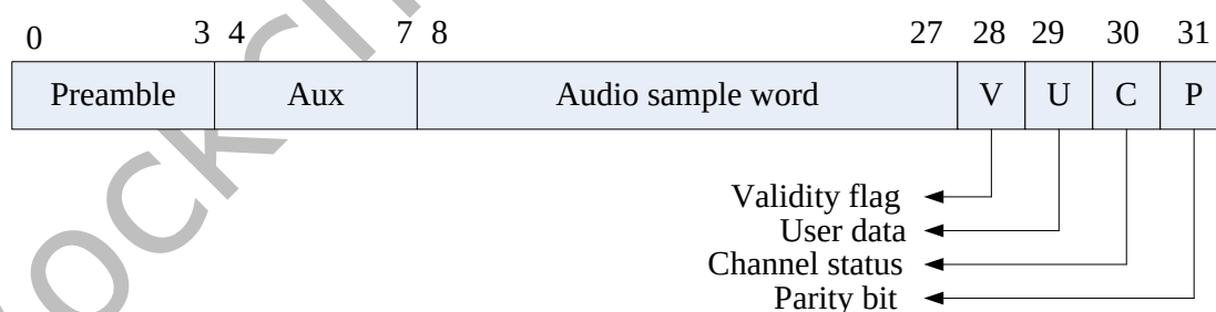
Fig. 14-3 SPDIF Sub-frame Format
